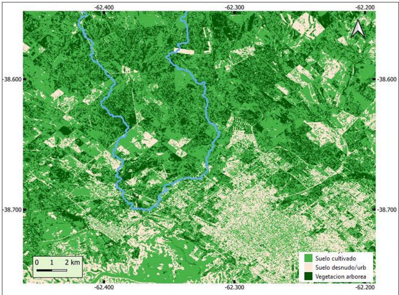
Figura 2. Clasificación por cobertura del suelo. Elaboración propia. Fuente QGIS 3.28
