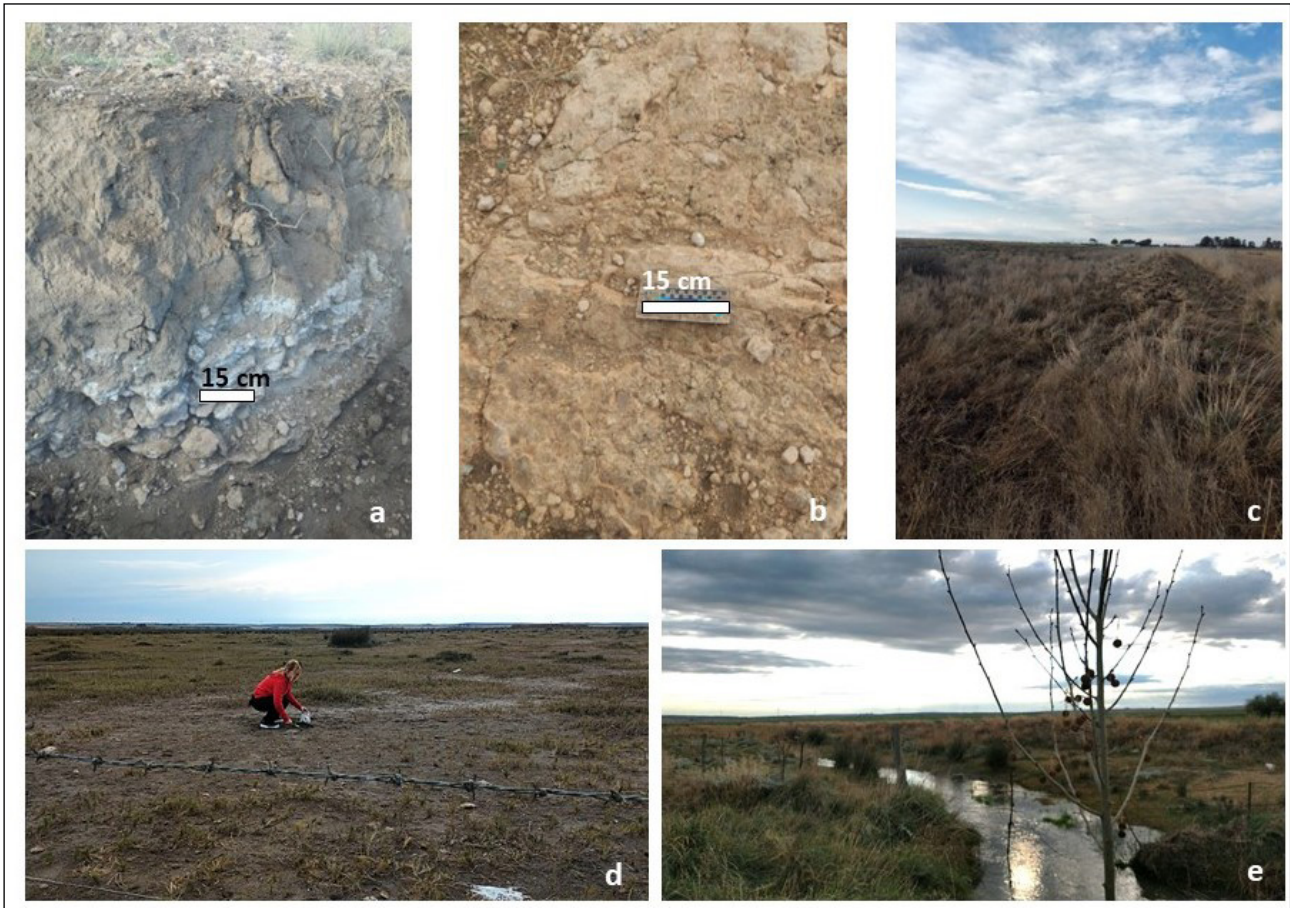
Figura 6. a) Calicata en punto de muestreo 1. b) Material aflorante de la Peniplanicie, M3. c y d) Llanura aluvial. e) Arroyo Saladillo, sector depósitos de valle fluvial.
