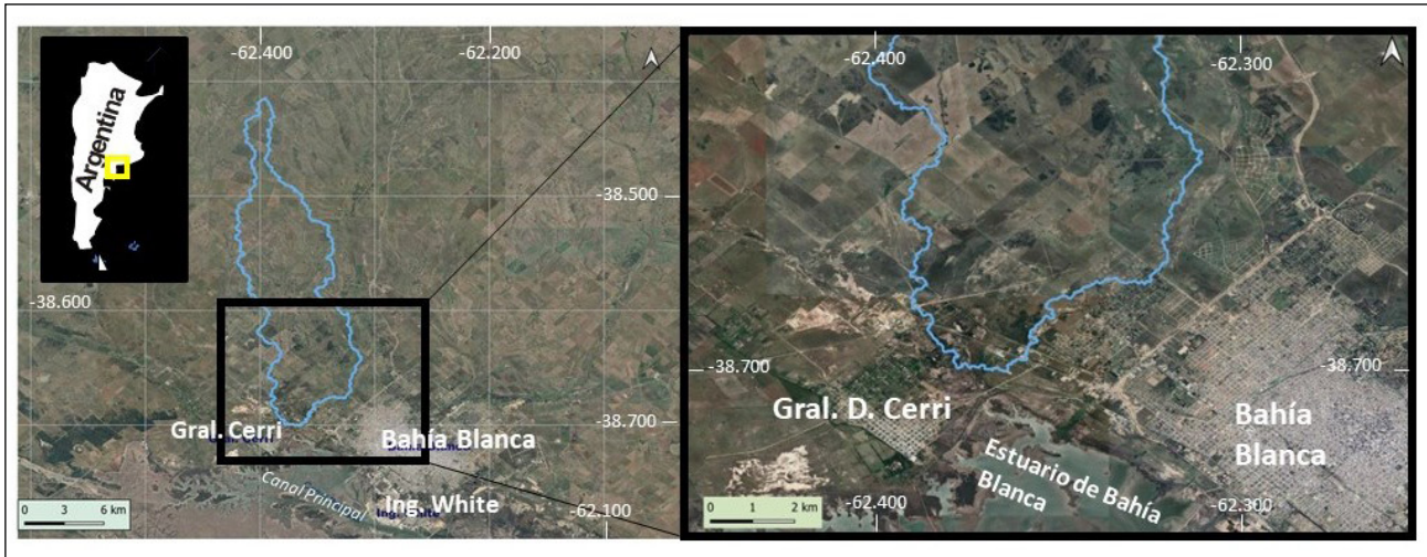
Figura 1. Localización del área de estudio. Delimitación de la cuenca de estudio. Elaboración propia. Fuente QGIS 3.28
