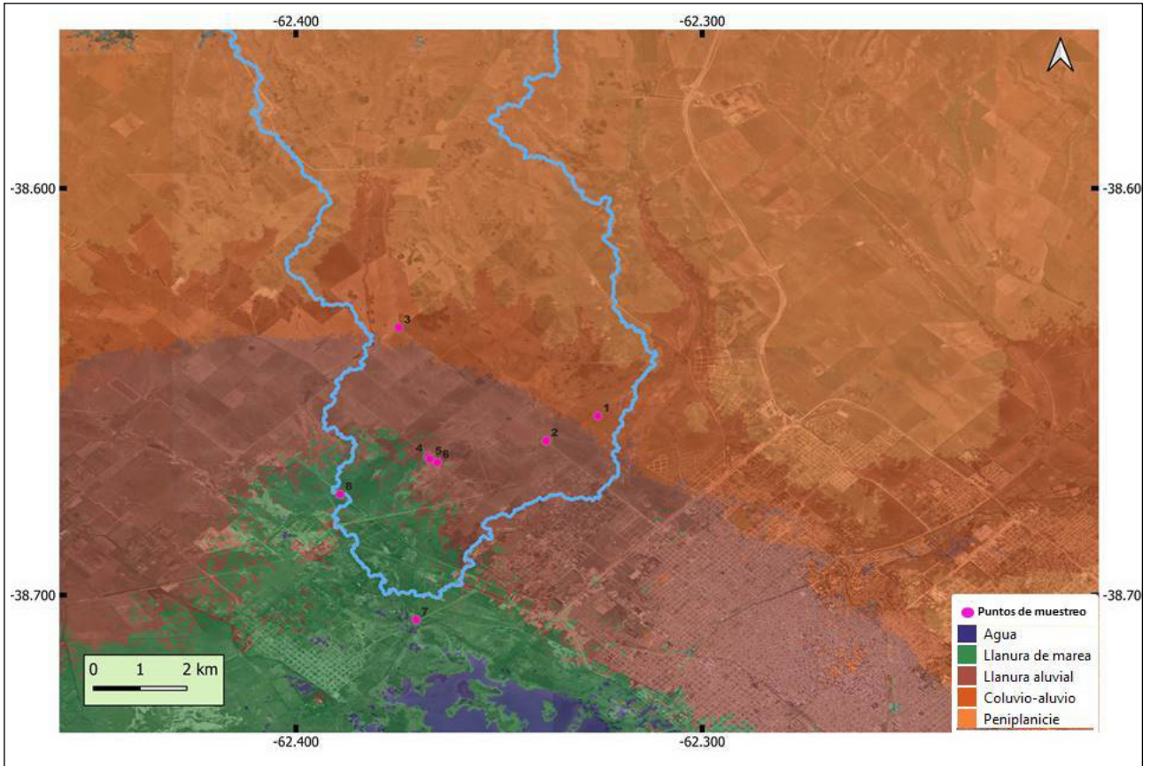
Figura 4. Unidades Geomorfológicas y puntos de muestreo sedimentológico. Elaboración propia. Fuente QGIS 3.28
