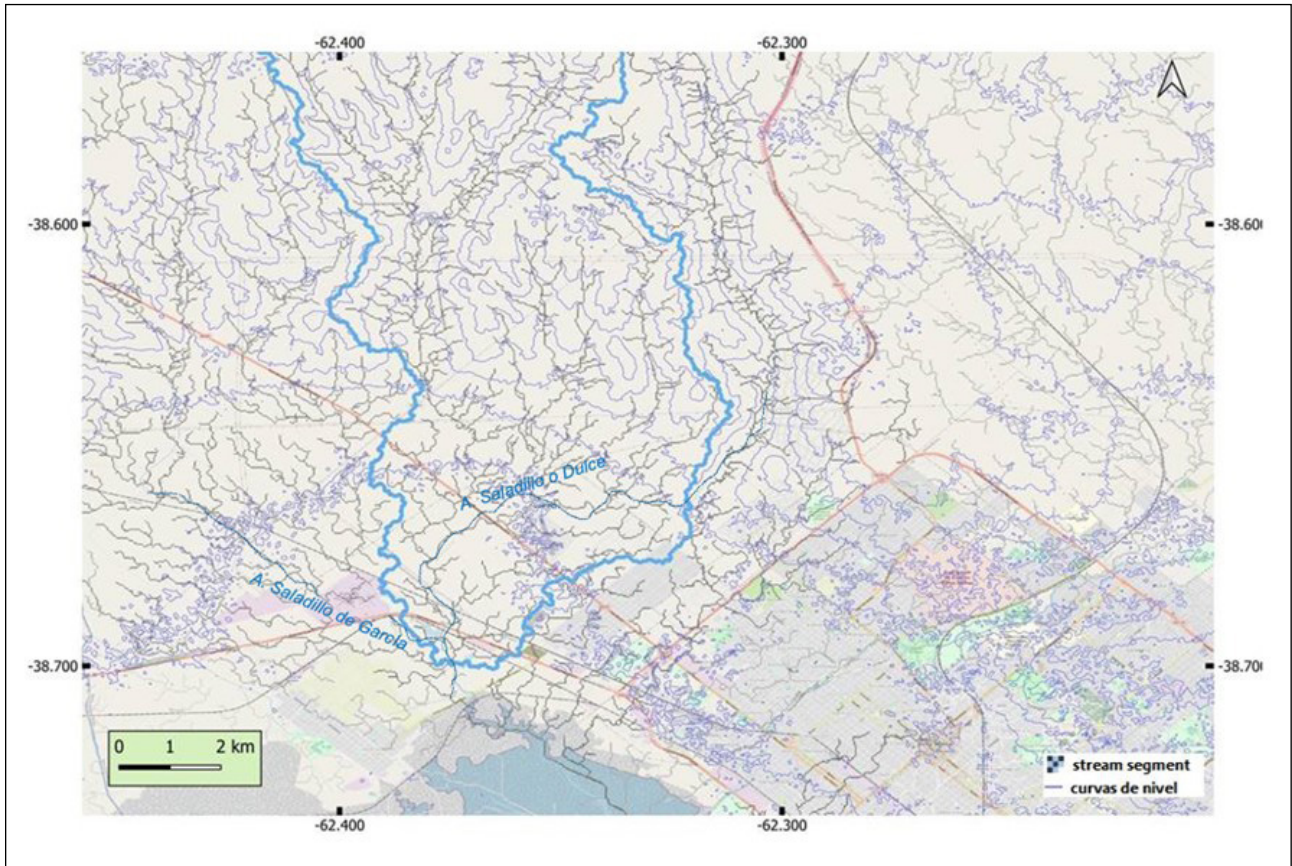
Figura 3. Curvas de nivel y red de drenaje. Elaboración propia. Fuente QGIS 3.28
