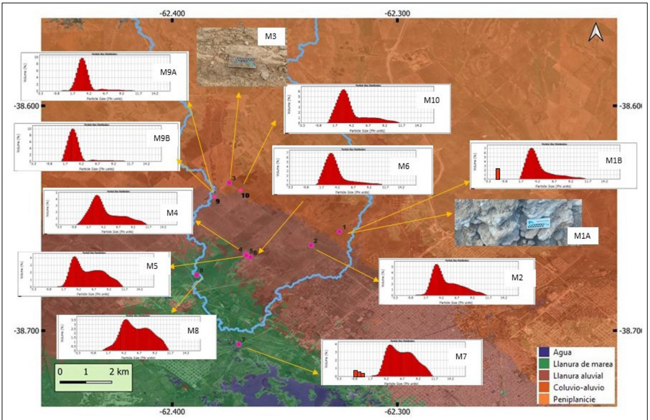
Figura 5. Localización de los puntos de muestreo y curvas de frecuencia de los sedimentos. Ubicación de los materiales consolidados estudiados.
