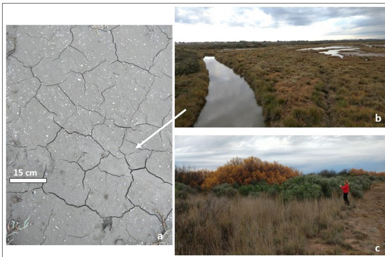
Figura 7. a) Vista en planta de la Planicie de marea emergida. b) Planicie de marea emergida surcada por un canal fluvio-marino. c) Área con sustrato de material removido y de relleno.
