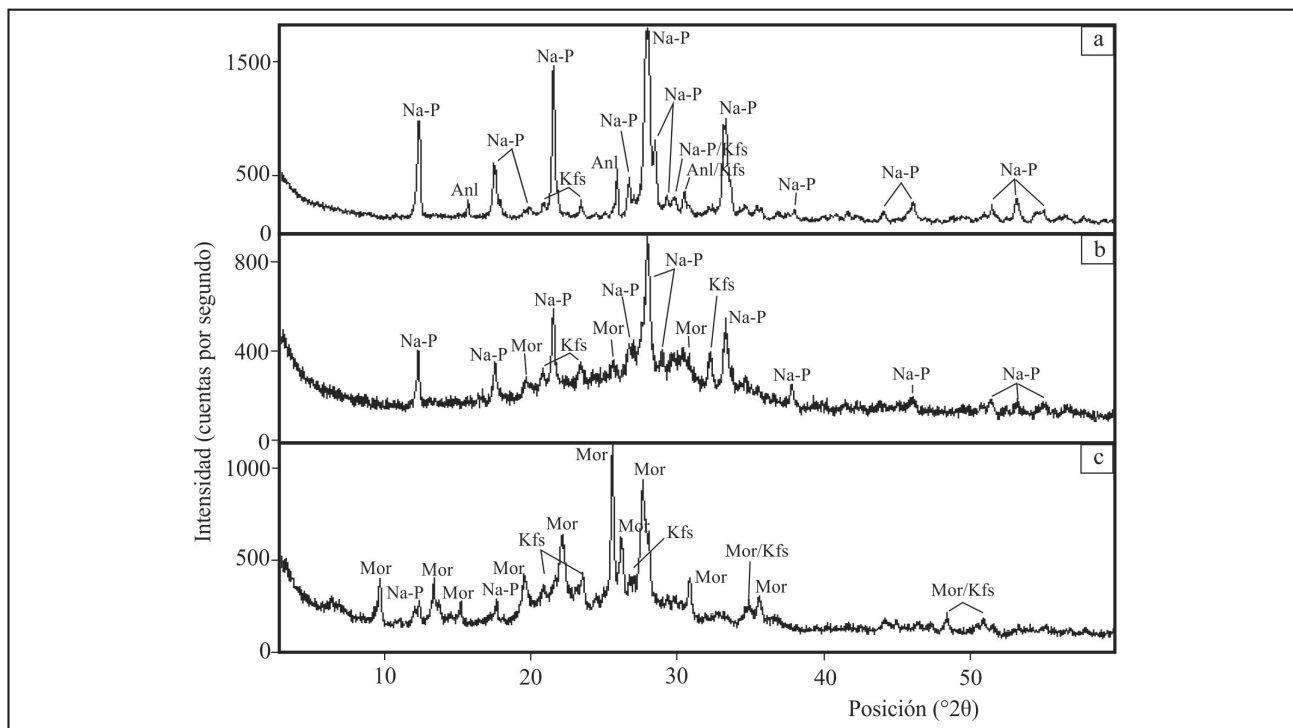
Figura 4. Difractogramas del material obtenido en los ensayos a 95 °C durante 4 semanas. a: con NaOH 1N. b: con NaOH 0,5 N. c: con NaOH 0,1 N. Mor: mordenita, Kfs: feldespato potásico, Na-P: zeolita Na-P, Anl: analcima.
