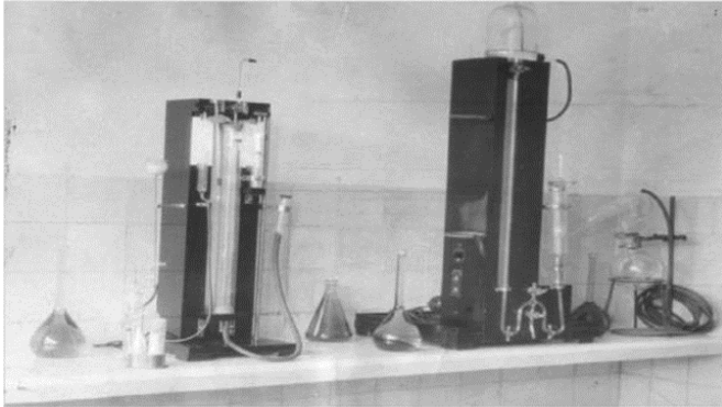
Figura 1. Instrumental del Instituto Ferreyra de 1951.
