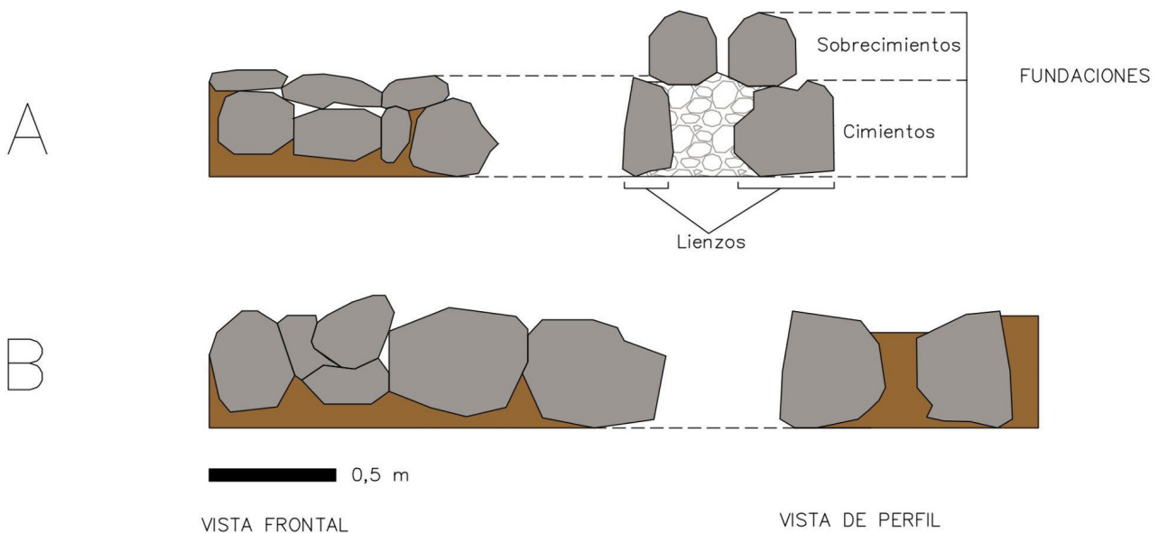
Figura 3. Detalle de vistas frontales y perfil de muros de A. R1 y B. R7
