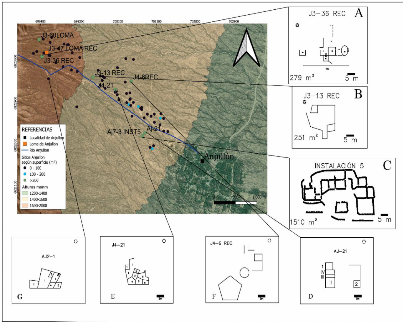
Figura 4. Planimetría de sitios mayores a 200 m 2 .
