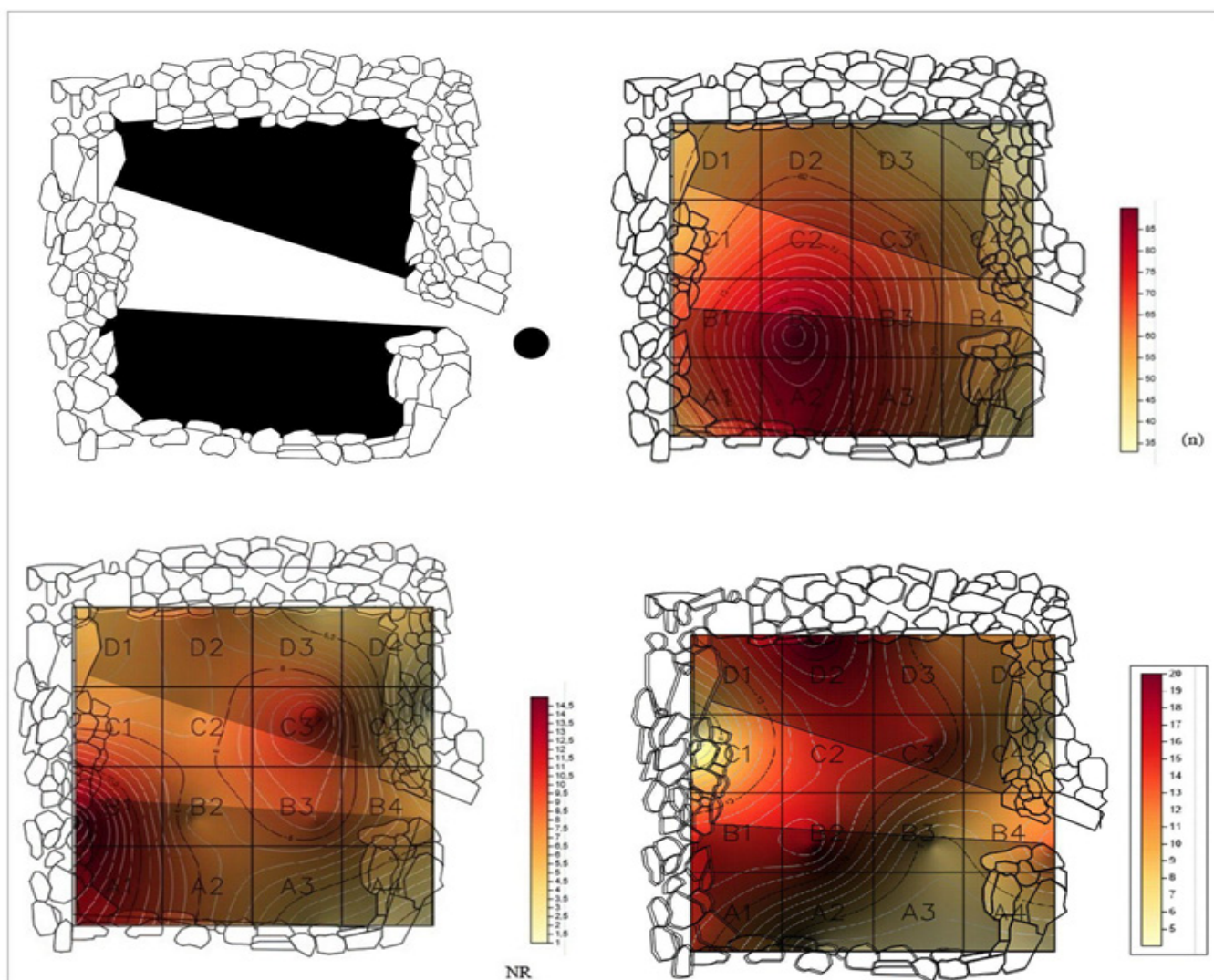
Figura 8. Kriging de concentración de materiales por cuadrícula. a) Área visible desde el exterior; b) Concentración material cerámica; c) Concentración materiales óseos; d) Concentración material lítico.
