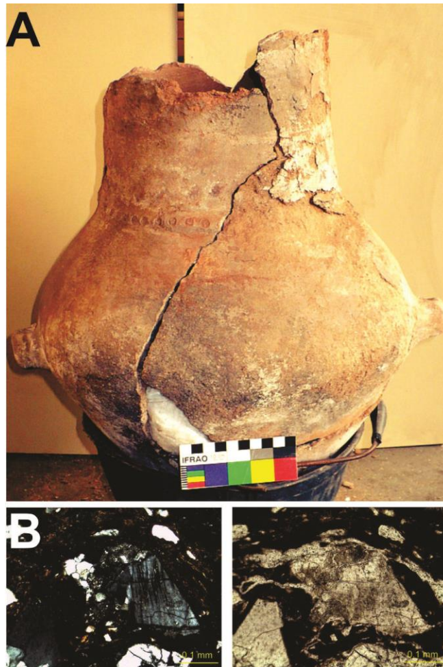
Figura 3: A. Fotografía de la Pieza 2. Cortesía de Martel (2011). B. Fotomicrografía de la pasta cerámica.
