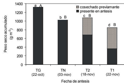
Figura 6: Biomasa acumulada hasta antesis de trigo con diferentes tratamientos de defoliación (Tabla 1). La fecha de antesis de cada tratamiento se presenta entre paréntesis. Letras iguales indican ausencia de diferencias significativas entre tratamientos ( p > 0,05 ), letras minúsculas marcan diferencias en la biomasa en antesis con una MDS de 295 g MS m -2 y letras mayúsculas en la biomasa acumulada con una MDS de 330 g MS m -2 .
