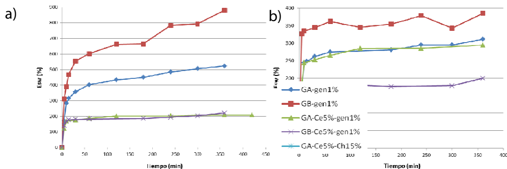
Figura 6. Índice de hinchamiento (%) en función del tiempo (min) de los films. a) pH = 3,5; b) pH = 6,8
