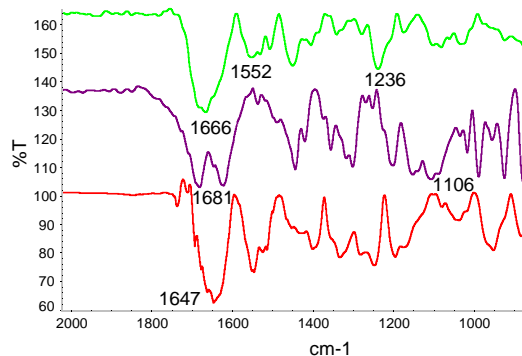
Figura 4. Espectros IR de GA5% (verde), genipín (azul) y GA5%-gen1% (rojo).
