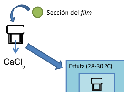
Figura 1. Equipo para la determinación de Permeabilidad.
