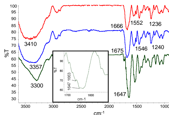
Figura 5. Espectros IR de GA5% (rojo), GA-Ce5% (azul) y GA-Ce5%-gen1% (verde).
